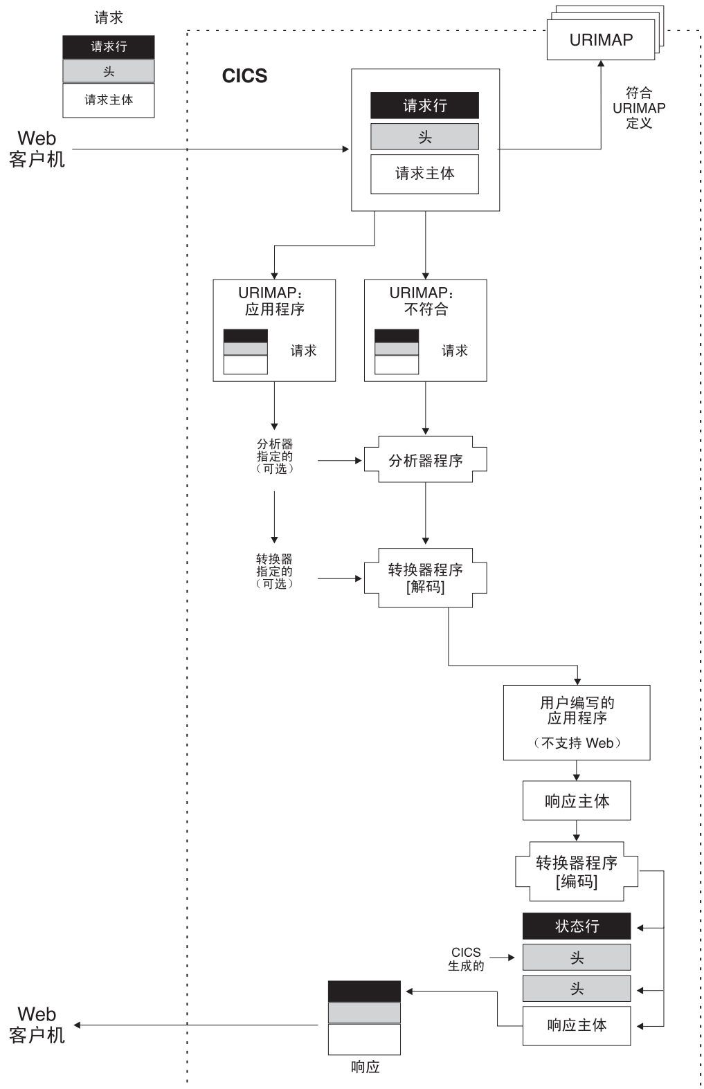
图 6. 来自通信区域应用程序的 HTTP 响应
