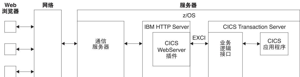
图 23. 处理来自 IBM HTTP Server 的请求
