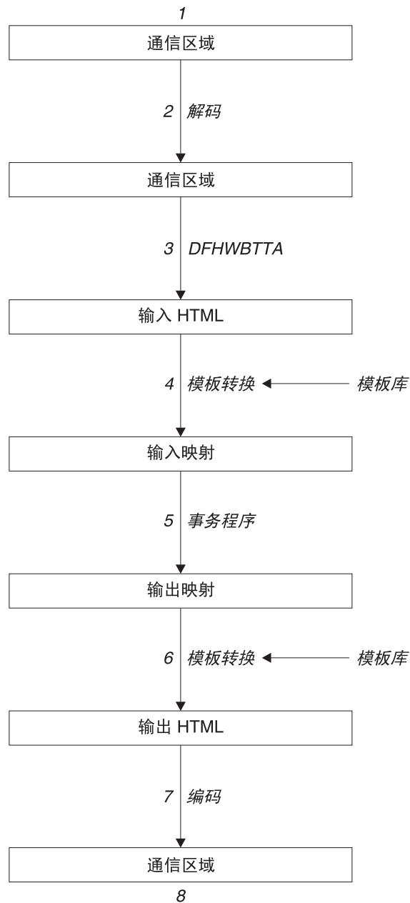
图 21. 继续面向终端的事务 - 数据流
