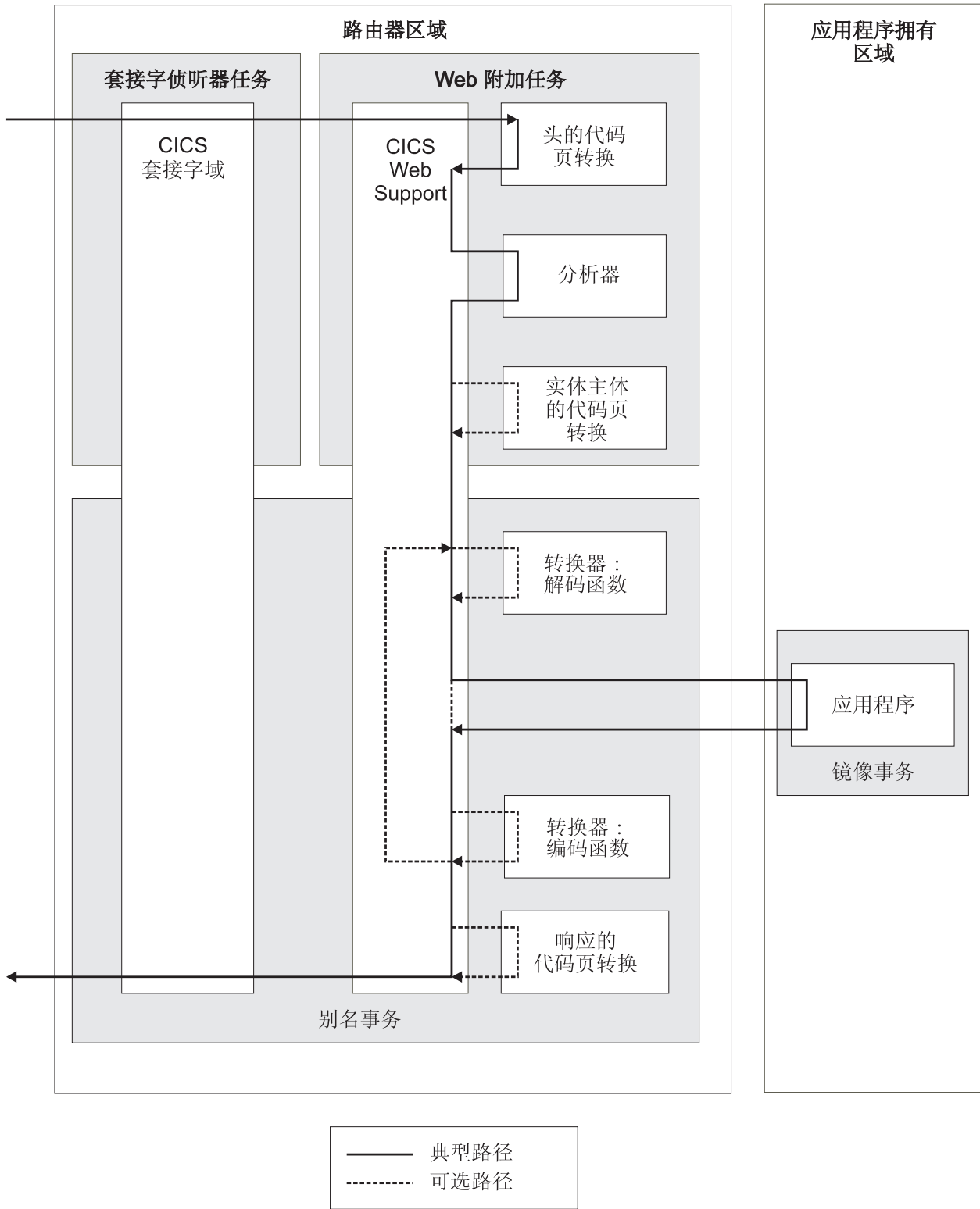
图 12. CICS Web Support 如何将非 Web 感知应用程序请求路由到 AOR
