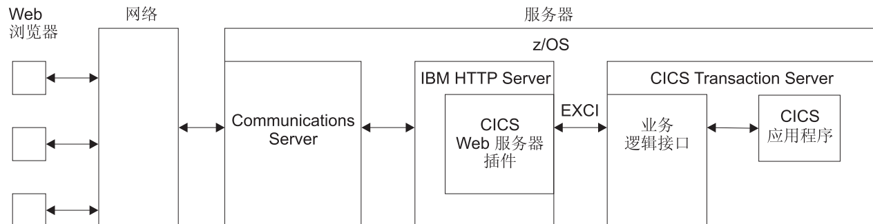
图 29. 处理来自 IBM HTTP Server 的请求
