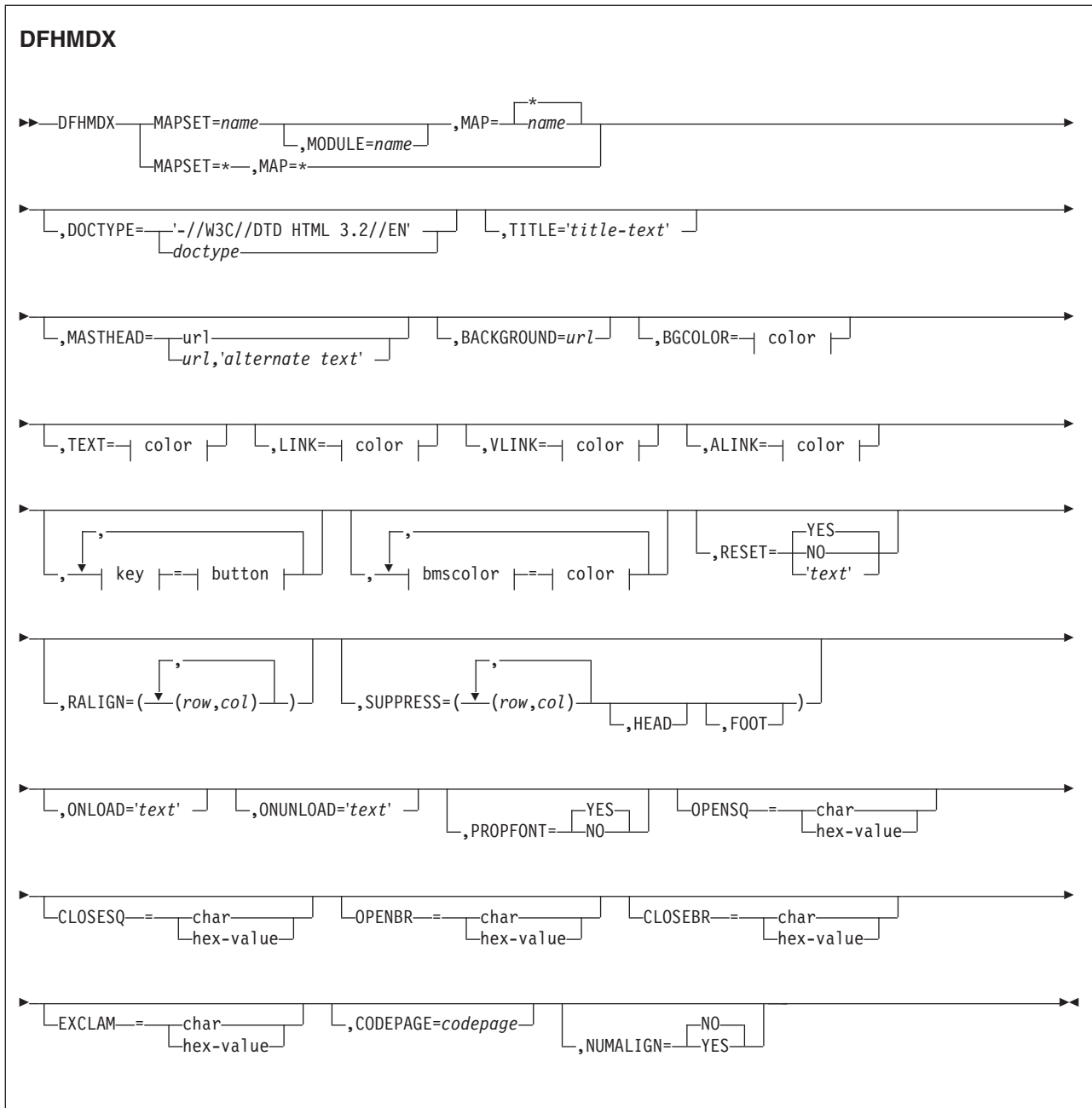
图 9. DFHMDX 的语法
