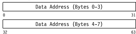
Format-2 IDAW
