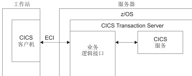
图 25. 处理 ECI 请求
