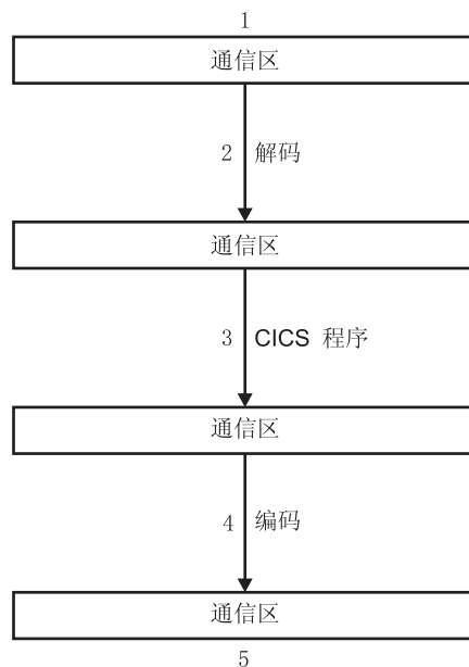
图 28. 用 CICS 业务逻辑接口调用程序 - 数据流
