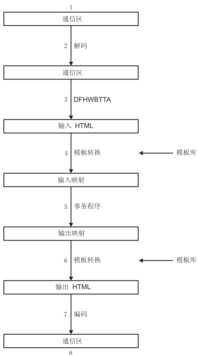
图 30. 继续面向终端的事务 - 数据流
