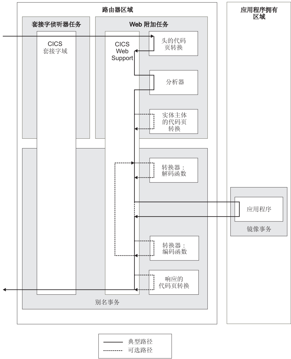
图 16. CICS Web Support 如何将非 Web 感知应用程序请求路由到 AOR
