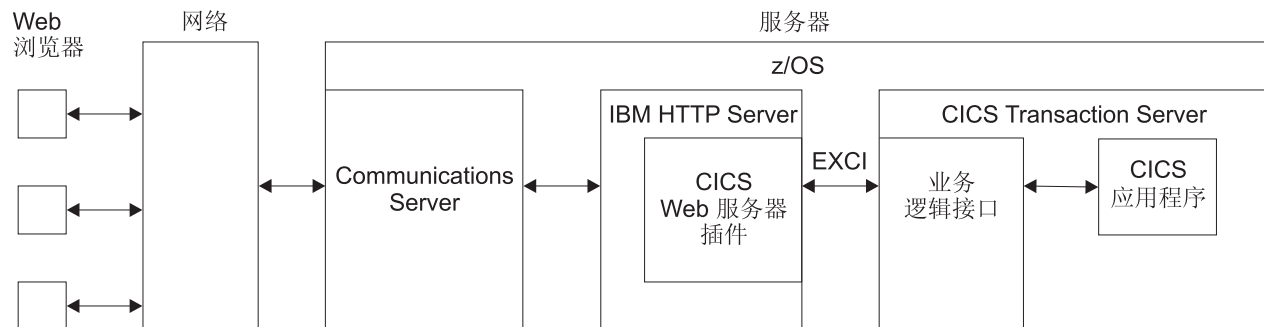
图 33. 处理来自 IBM HTTP Server 的请求
