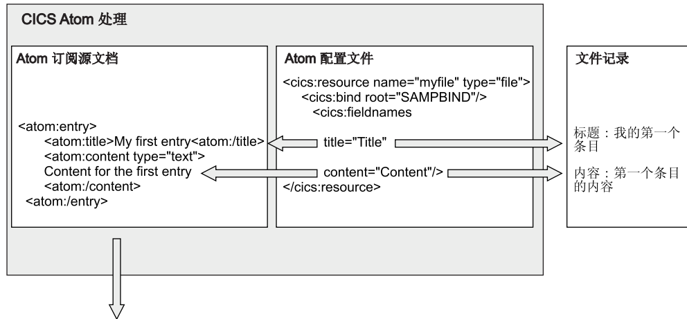
图 18. 直接从文件中抽取 Atom 条目数据
