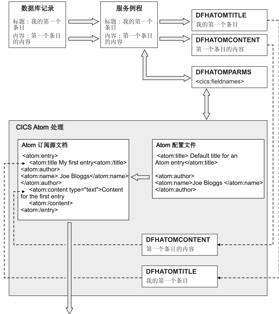
图 19. 使用服务例程提供 Atom 条目数据
