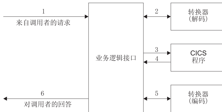
图 26. 用 CICS 业务逻辑接口调用程序 - 控制流
