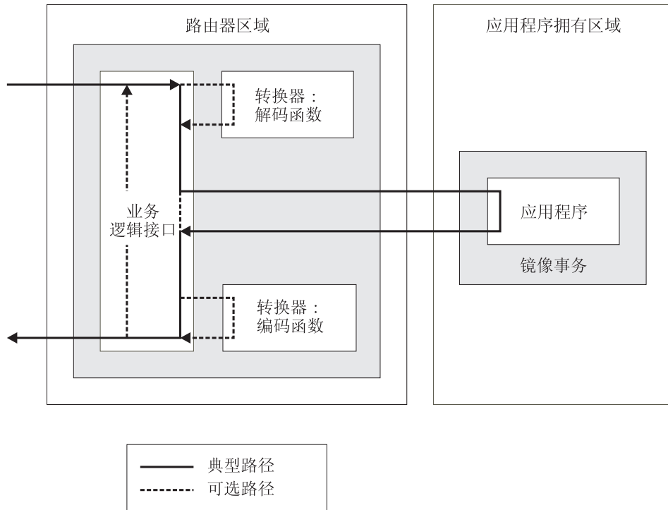
图 17. CICS 业务逻辑接口如何将应用程序请求路由到 AOR
