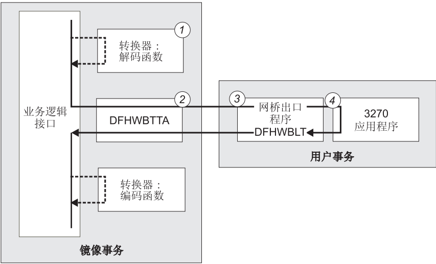
图 27. 用 CICS 业务逻辑接口运行事务 - 控制流
