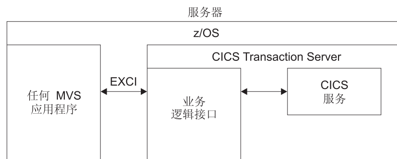
图 24. 处理 EXCI 的请求
