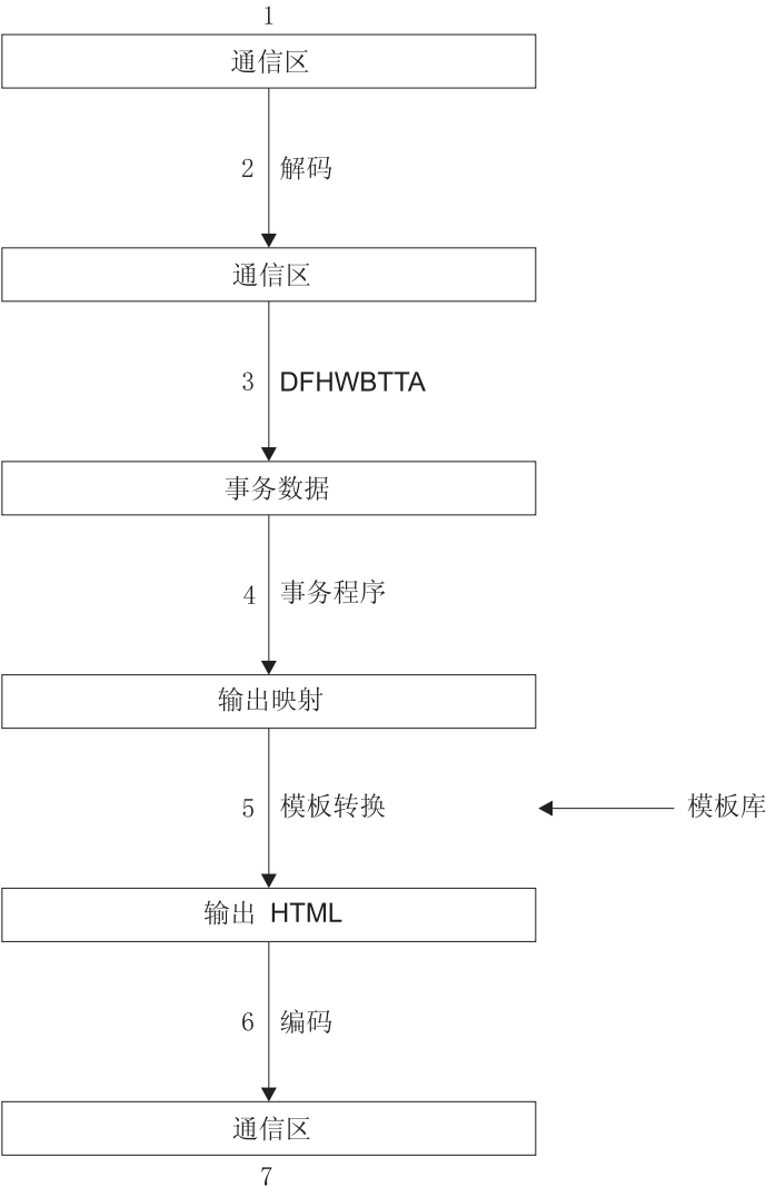
图 29. 启动面向终端的事务 - 数据流
