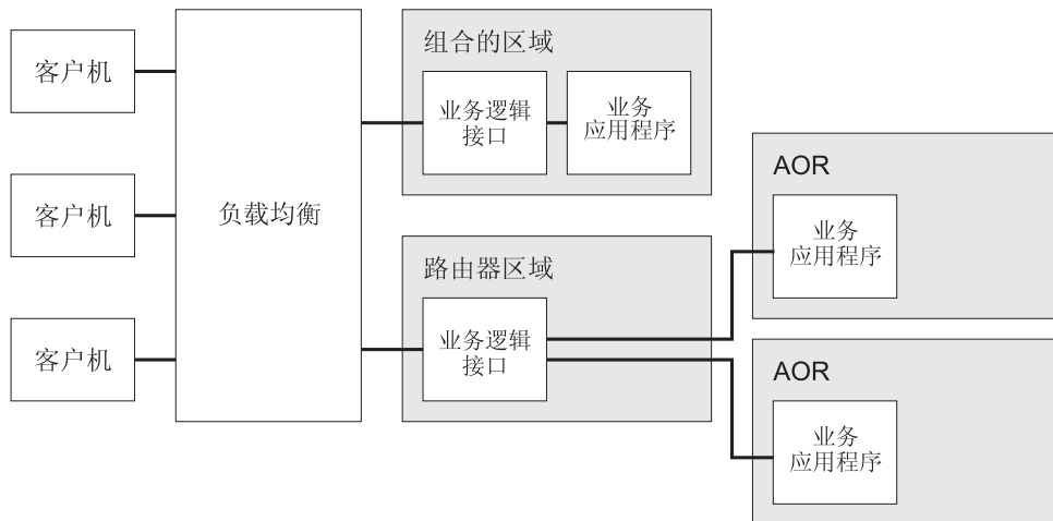
图 15. CICSplex 中的 CICS 业务逻辑接口配置
