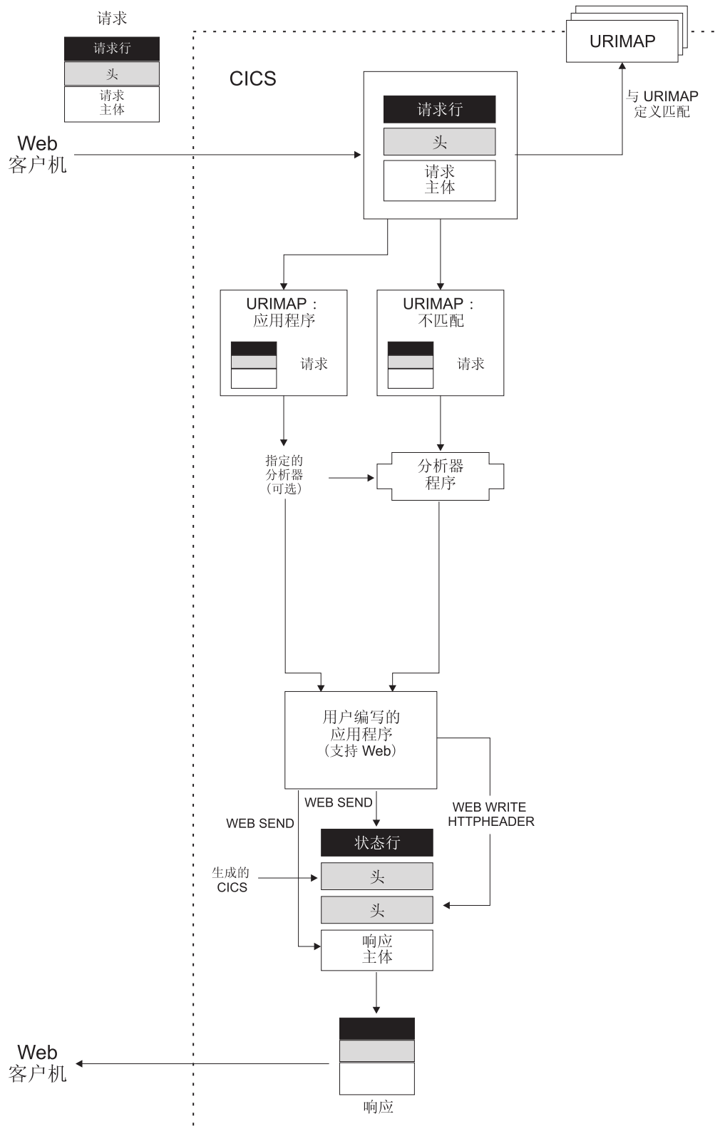
图 4. 使用 Web 感知应用程序提供的动态 HTTP 响应
