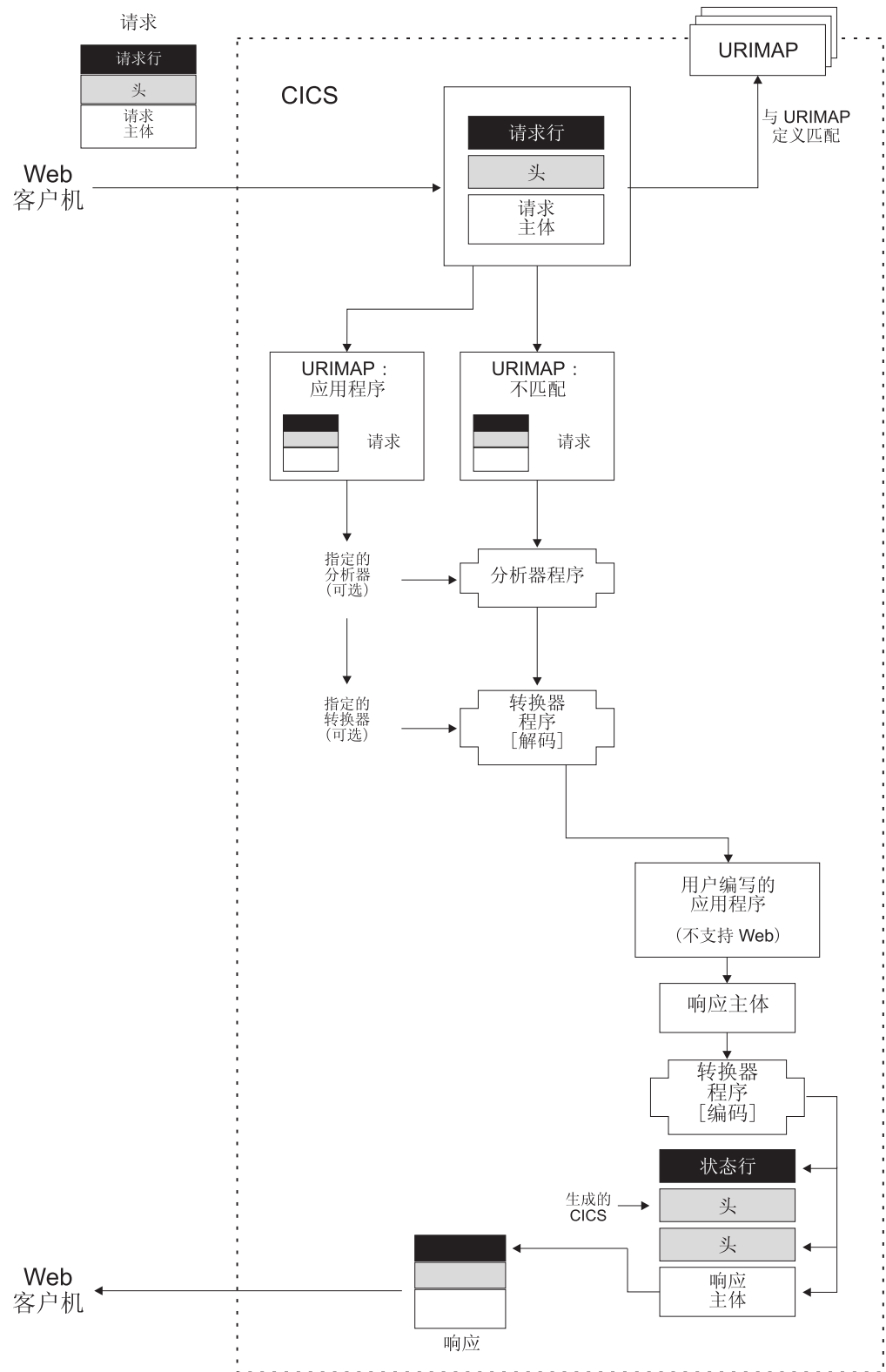
图 6. 来自 COMMAREA 应用程序的 HTTP 响应
