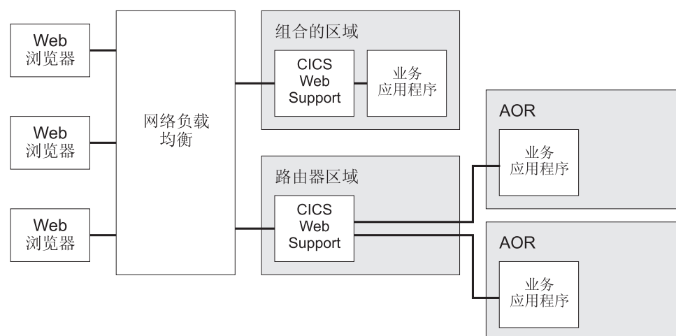
图 7. CICSplex 中的 CICS Web Support 配置
