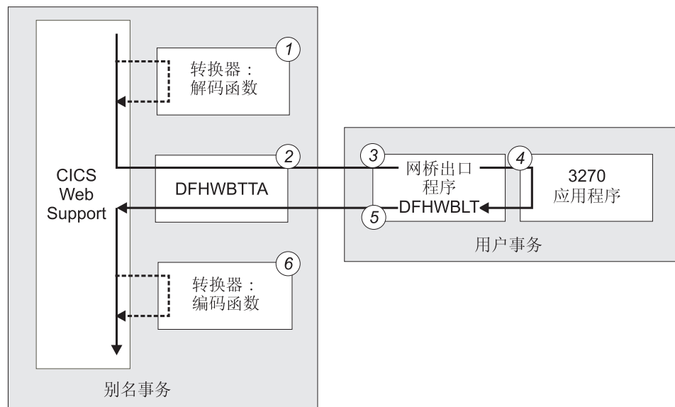
图 11. CICS Web Support 如何与 3270 应用程序交互
