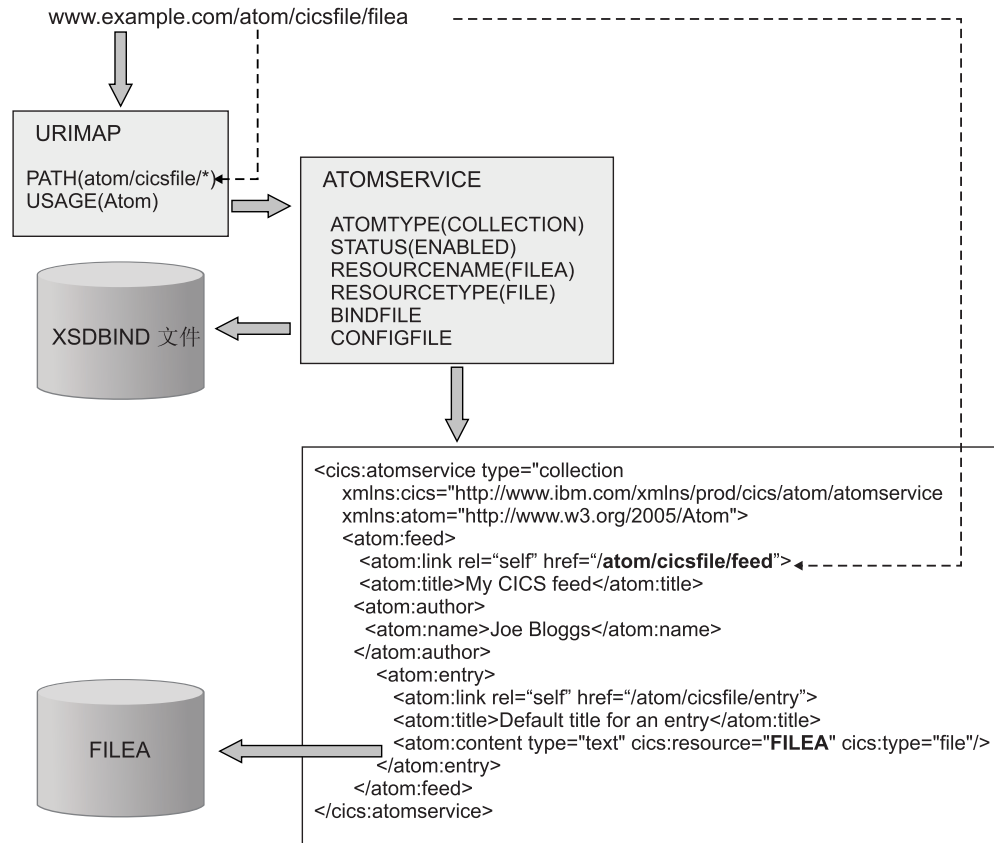
图 20. Atom 订阅源的请求 URL
