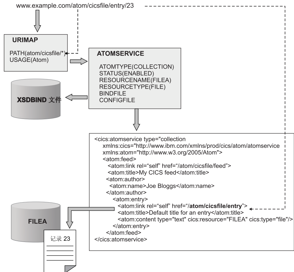
图 21. 针对 Atom 条目的请求 URL
