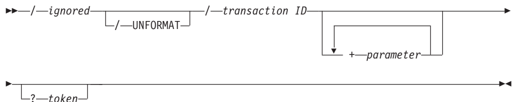
图 12. DFHWBTTA 解释的路径语法
