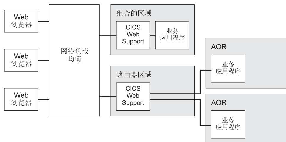
图 14. CICSplex 中的 CICS Web Support 配置
