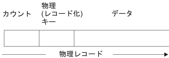
図 119. BDAM データ・セットの非ブロック化レコードの形式
