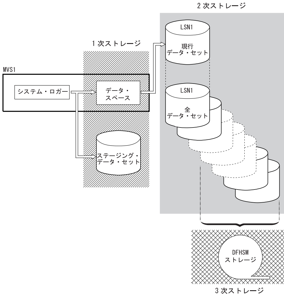
図 10. MVS システム・ロガーで使用されるストレージのタイプ： この図は、ストレージ専用ロギングを使用するログ・ストリームを示しています。1 次ストレージは、システム・ロガーと同じ MVS イメージ内のデータ・スペースと、単一ステージング・データ・セットから構成されます。2 次ストレージは、単一ステージング・データ・セットの連続するコピーを保持するディスク装置上の一連のデータ・セットから構成されます。3 次ストレージは、古いレベルの 2 次ストレージ・データ・セットを保持する DFHSM ストレージです。
