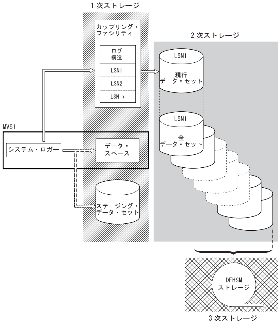
図9. MVS システム・ロガーで 사용되는ストレージのタイプ： この図は、カップリング・ファシリティを使用するログ・ストリームを示しています。1 次ストレージは、カップリング・ファシリティ内の構造のスペースと、システム・ロガーと同じ MVS イメージ内のステージング・データ・セットまたはデータ・スペースのいずれかのスペースから構成されます。2 次ストレージは、カップリング・ファシリティ内のログ構造の元素がマップされるディスク装置上の一連のデータ・セットから構成されます。3 次ストレージは、古いレベルの 2 次ストレージ・データ・セットを保持する DFHSM ストレージです。
