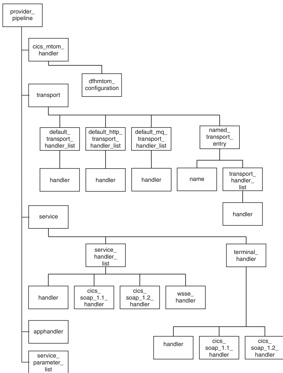
図 21. サービス・プロバイダーのパイプライン定義の構造 :
