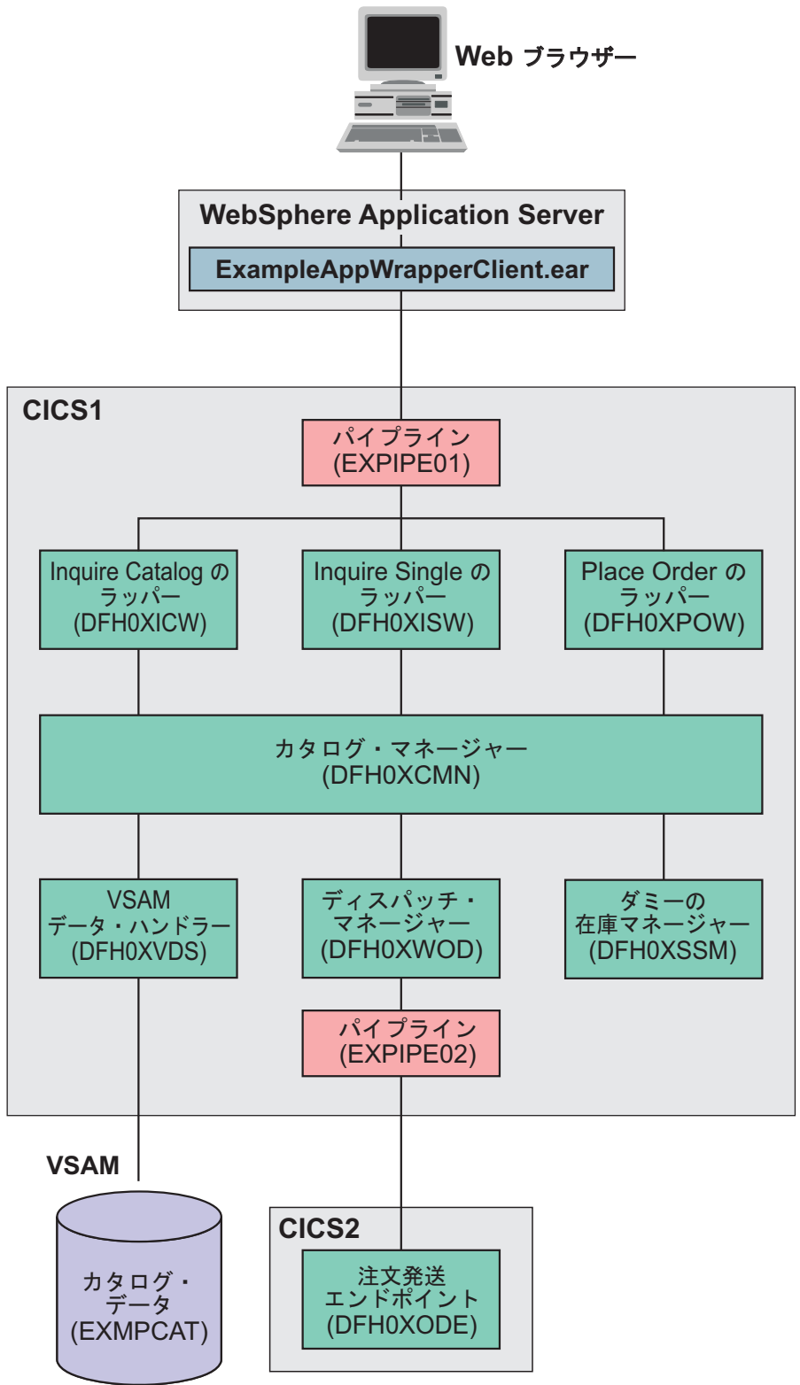
図 30. 代替の Web サービス・プロバイダー構成
