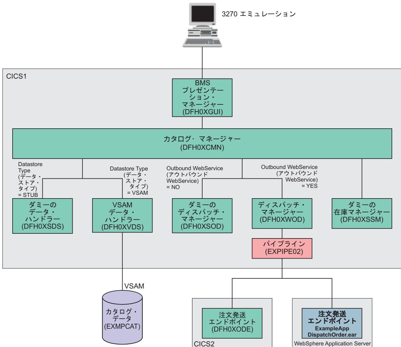
図 28. ベース・アプリケーションの構造
