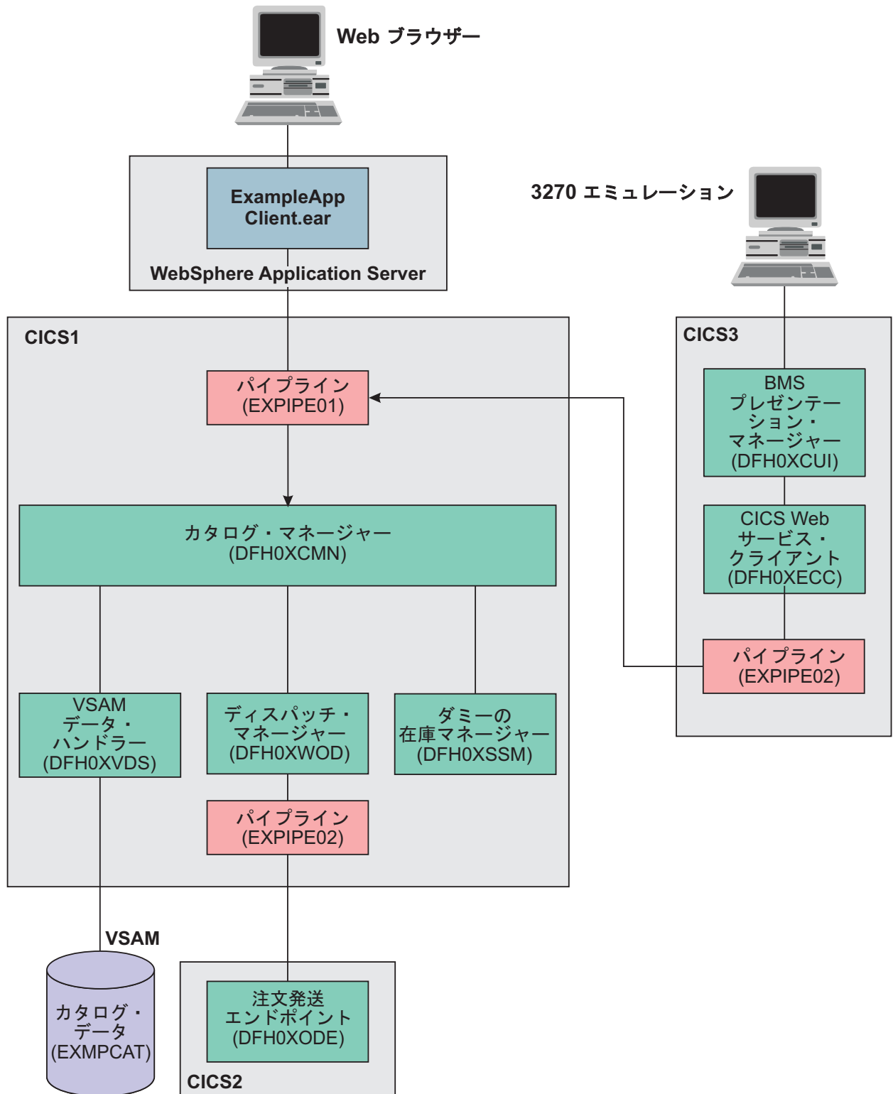
図 29. Web サービス・プロバイダーとして構成された実例アプリケーション
