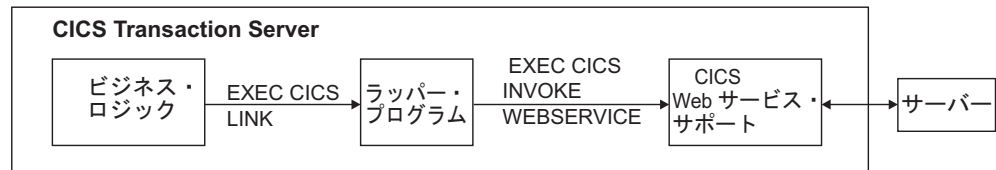
図 20. ラッパー・プログラム使用による、Web サービス・リクエスターとしての CICS アプリケーションの配置
