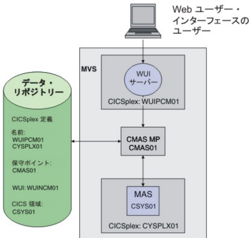
図 11. 単純な CICSplex SM 環境
