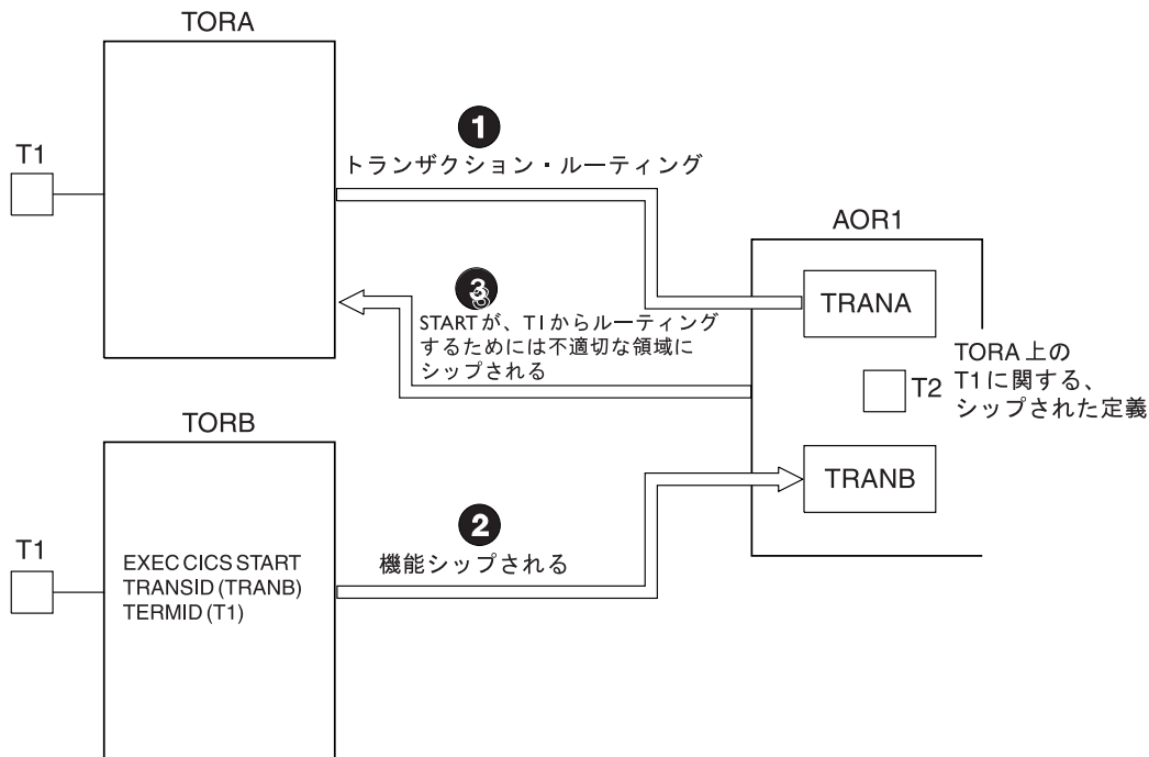
図 24. 正しくない端末に対して開始される機能シップされた START 要求： 端末 T1 (TORA によって所有される) のシップされた定義は AOR1 にインストールされていますので、TORB から受信された START 要求は、ルーティングに対し、TORB ではなく TORA へシップされます。
