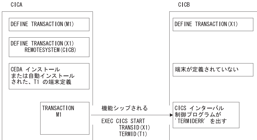
図 22. 端末 ID が認識されていないシステムでの ATI 要求の失敗
