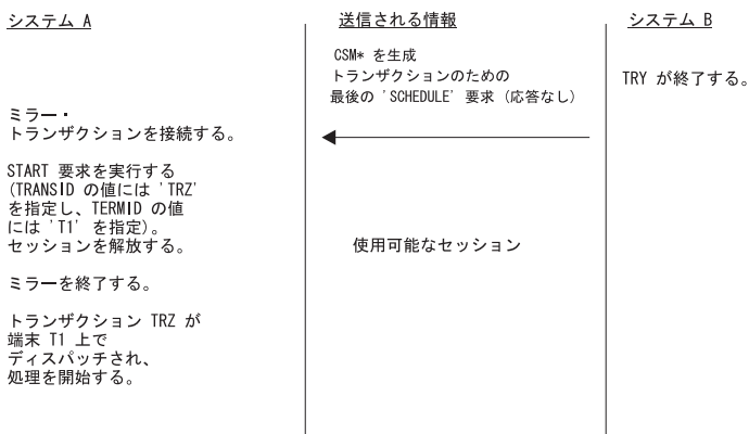
図 17. 非同期処理 - NOCHECK を使用したリモート・トランザクションの開始：この例は、ISC 接続、または長期実行ミラーのない MRO 接続を示しています。
