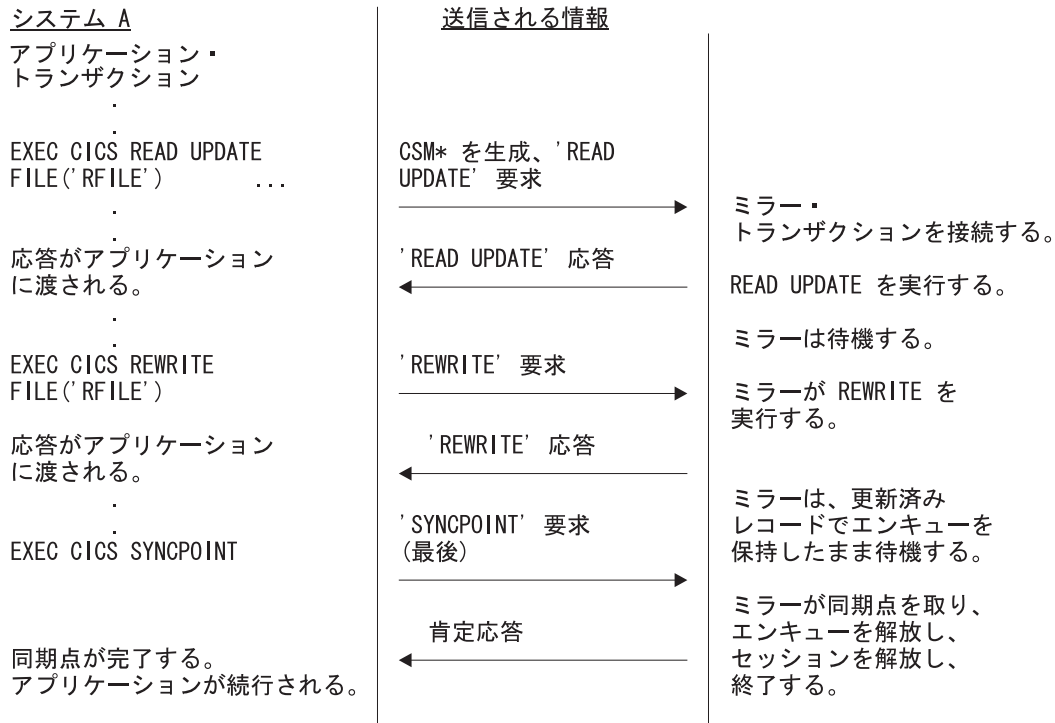
図 13. ISC または MRO 機能シップ - 更新: ミラーは、REWRITE まで待機しなければならないため長期実行タスクとなり、SYNCPOINT を受け取るまで終了しません。ファイルがリカバリー可能でない限り、更新されたレコードでのエンキューは、REWRITE コマンドが終わった後は保持されないことに注意してください。
