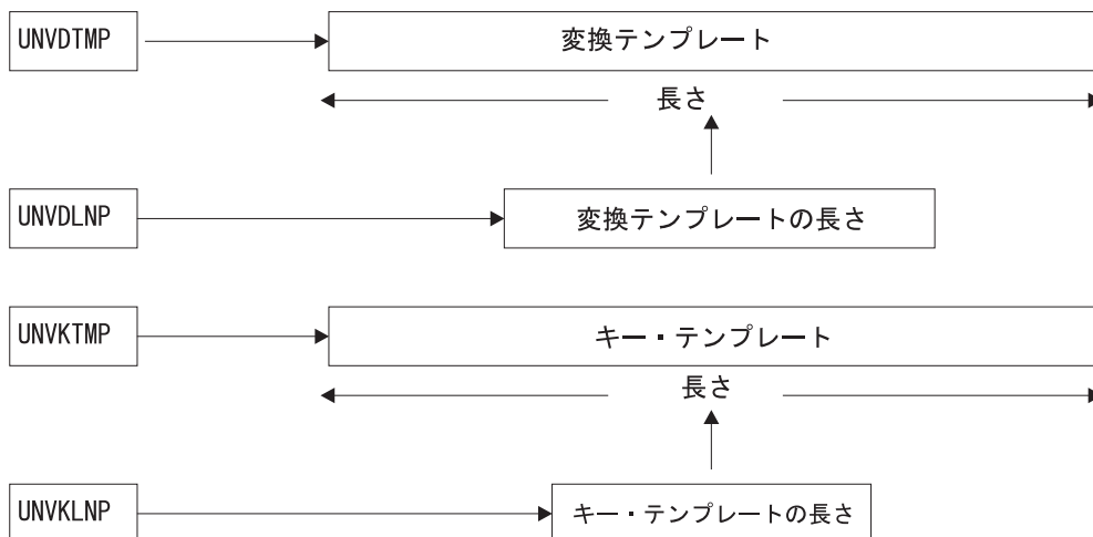
図 109. パラメーター・フィールドと変換テンプレート
