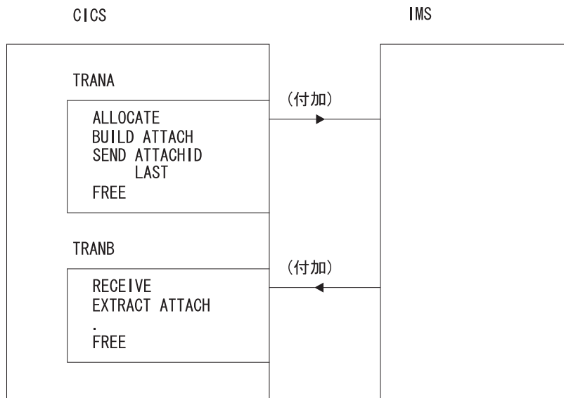
図 84. SEND と RECEIVE の非同期処理 - CICS フロントエンド
