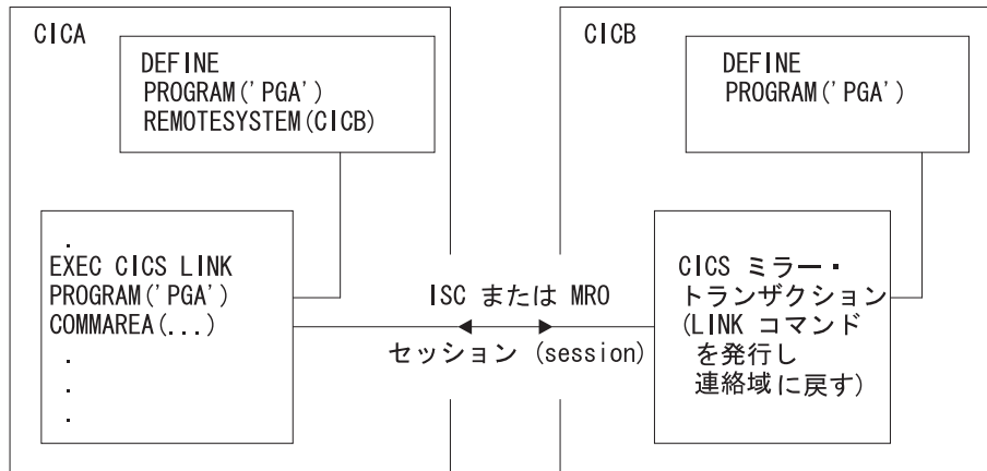
図 30. 分散プログラム・リンク
