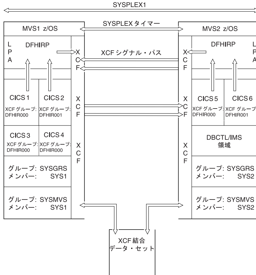
図7. 2 つの CICS XCF グループを含むシスプレックス (SYSPLEX1)
