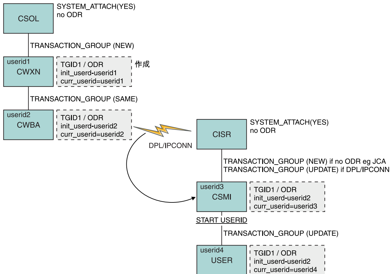
図 4. HTTP 要求が処理される際の発信元データの作成と移動
