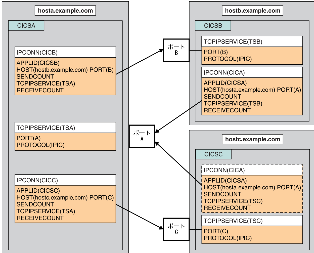
図3. 関連した IPCONN 定義と TCPIPService 定義
