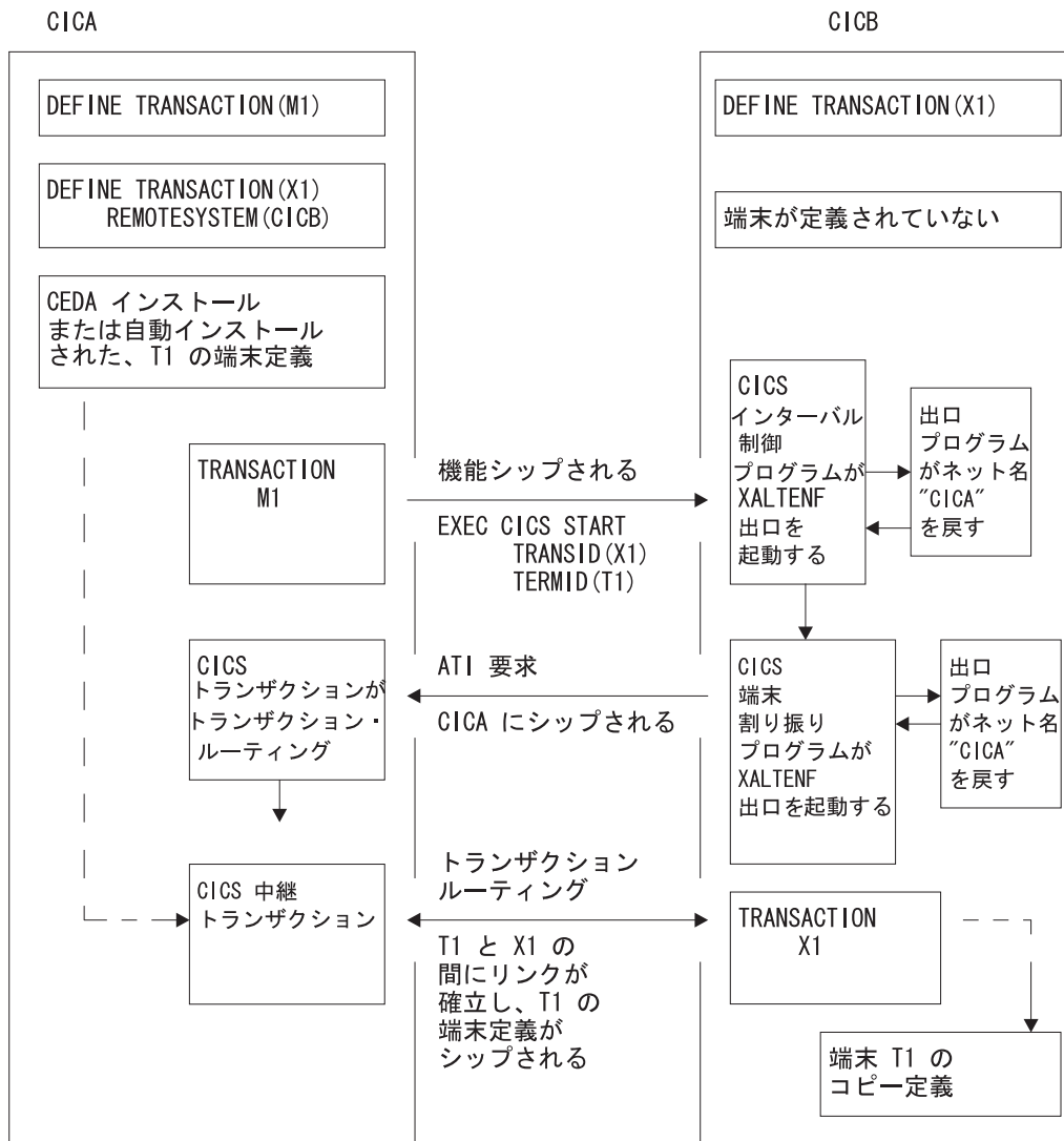
図 23. START 要求における「端末未認識」状態の解決
