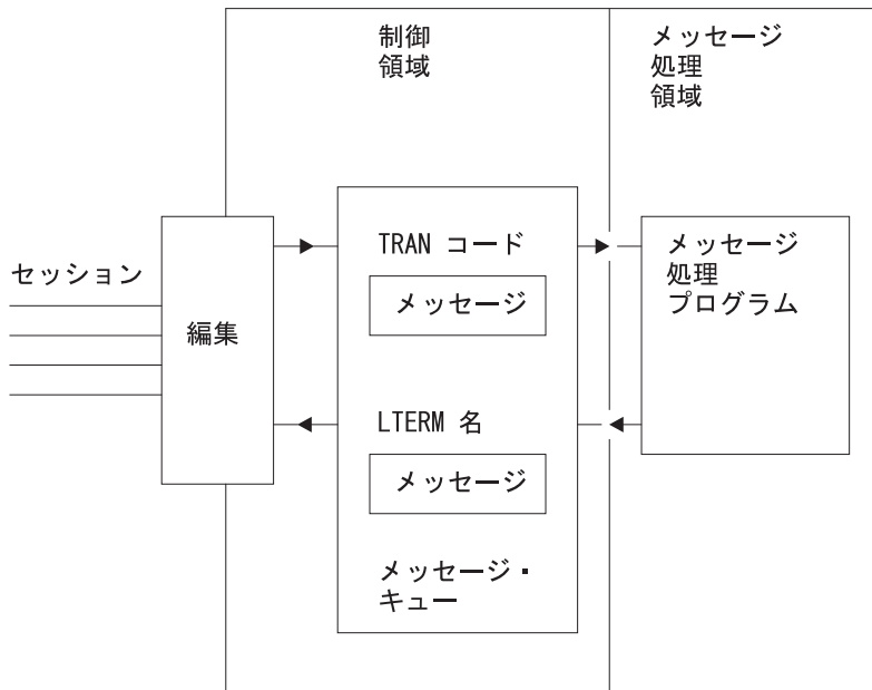
図 81. 基本的な IMS メッセージ・キュー化
