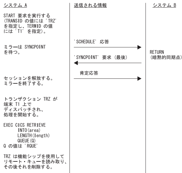
図 16. 非同期処理 - リモート・トランザクションの開始：この例では、長期実行ミラー (MROLRM) がシステム A に対しては指定されているが、システム B に対しては指定されていない MRO 接続を示します。2 つのシステムでのミラー・トランザクションのアクションの違いに注意してください。
