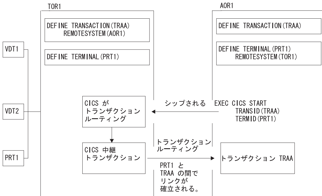
図 21. ATI によって開始されたトランザクション・ルーティング
