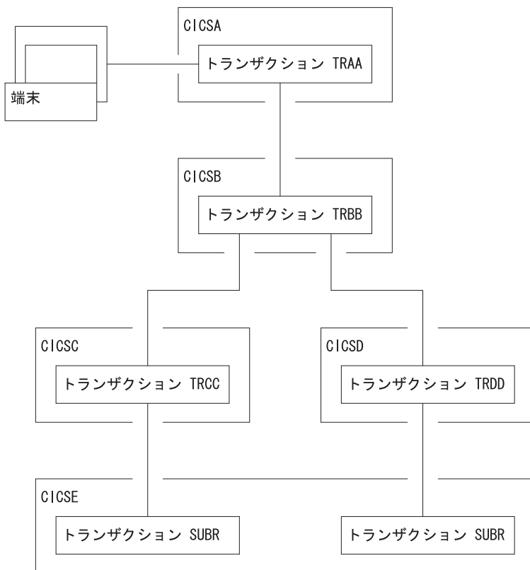
図 34. 複数システム構成の DTP
