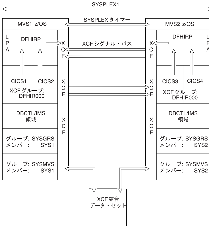
図6. 単一の CICS XCF グループを含むシスプレックス (SYSPLEX1) :
