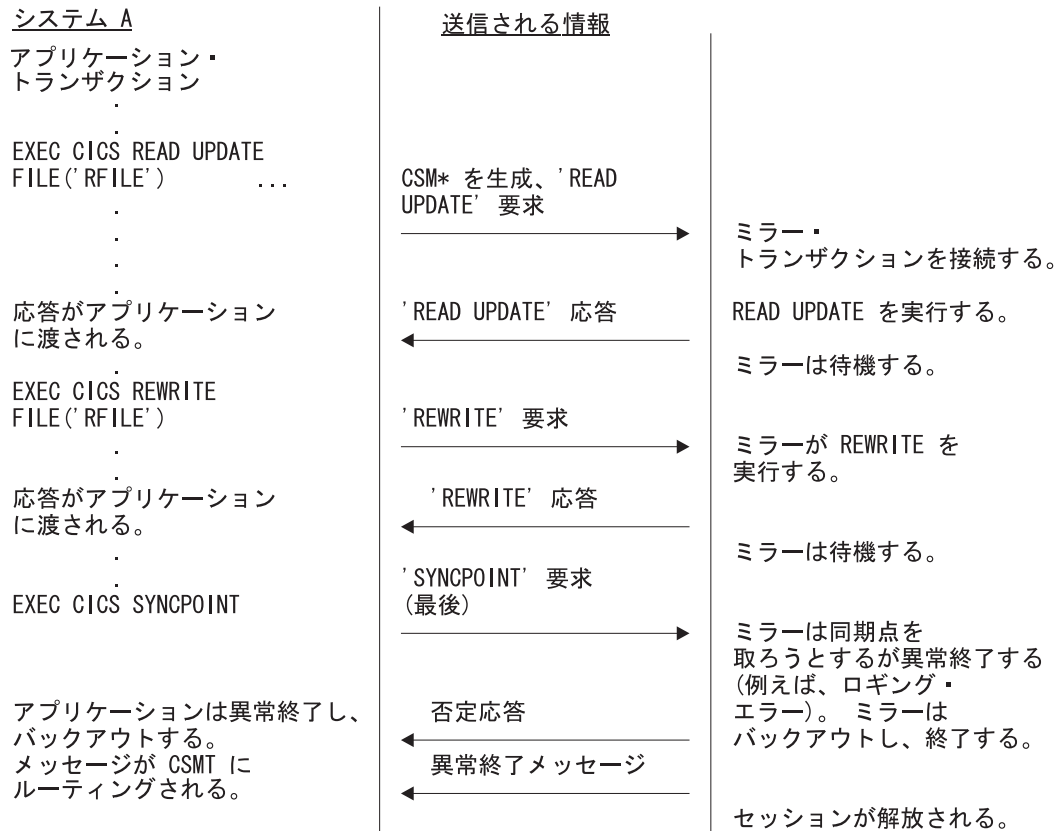
図 14. ISC または MRO 機能シップ - 更新 (ABEND)
