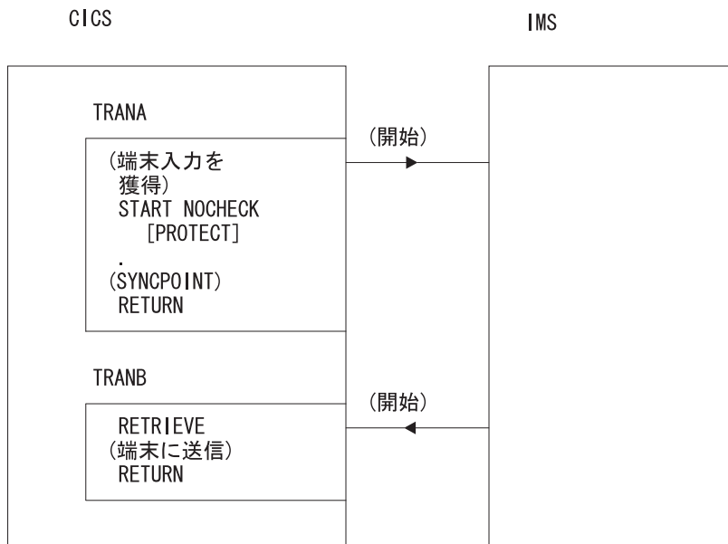
図 82. START と RETRIEVE の非同期処理 - CICS フロントエンド
