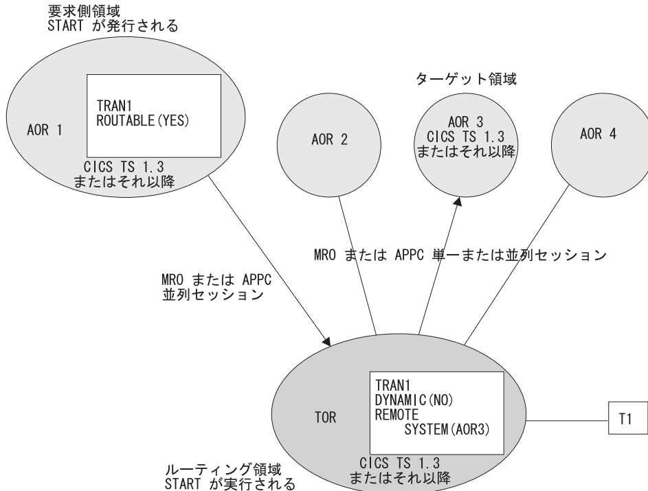
図 25. 拡張方法を使用した、AOR で発行された端末関連 START コマンドの静的ルーティング
