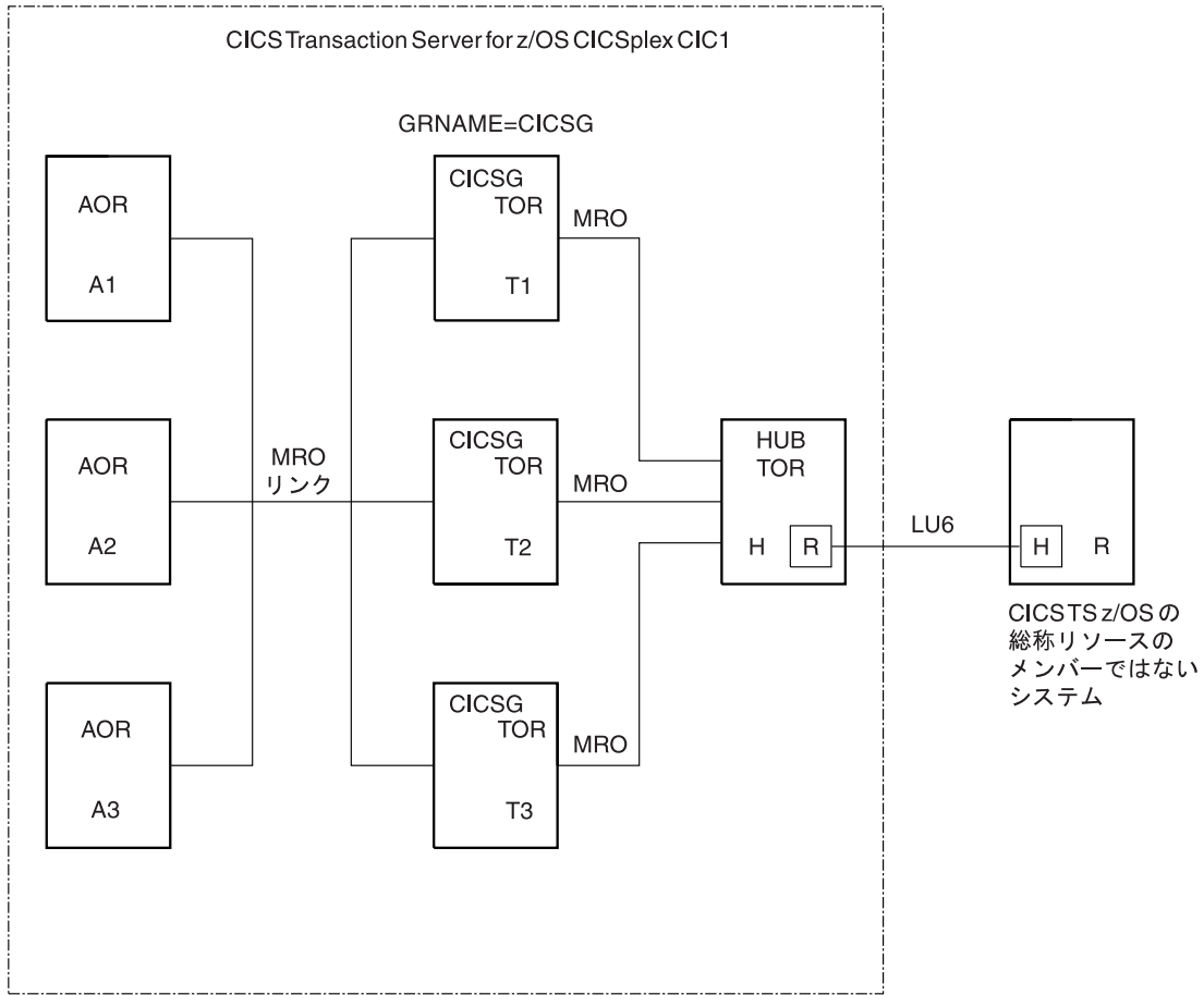
図 40. ネットワーク・ハブ： ハブは通常、総称リソース・グループのメンバーから、CICS Transaction Server for z/OS 総称リソースのメンバーではないシステムへのアウトバウンド LU6 要求に使用されます。
