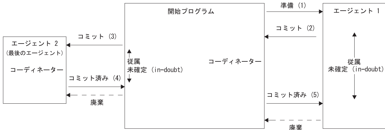
図 87. 同起点処理フロー - 複数セッション: この分散 UOW では、開始プログラムは、エージェント 1 のコーディネーターであると同時に、エージェント 2 の従属です。エージェント 2 は最後のエージェントですので、コミットの準備の通知は受けません。
