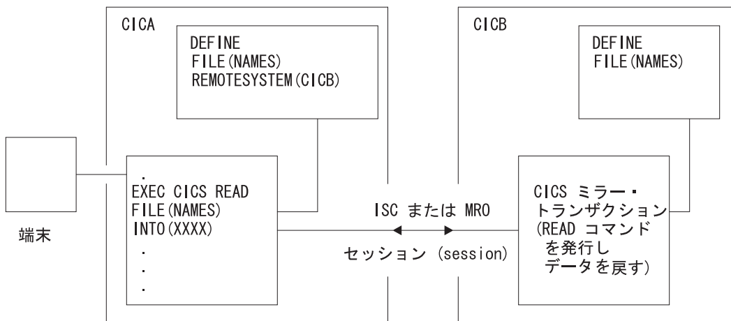
図 8. 機能シップ
