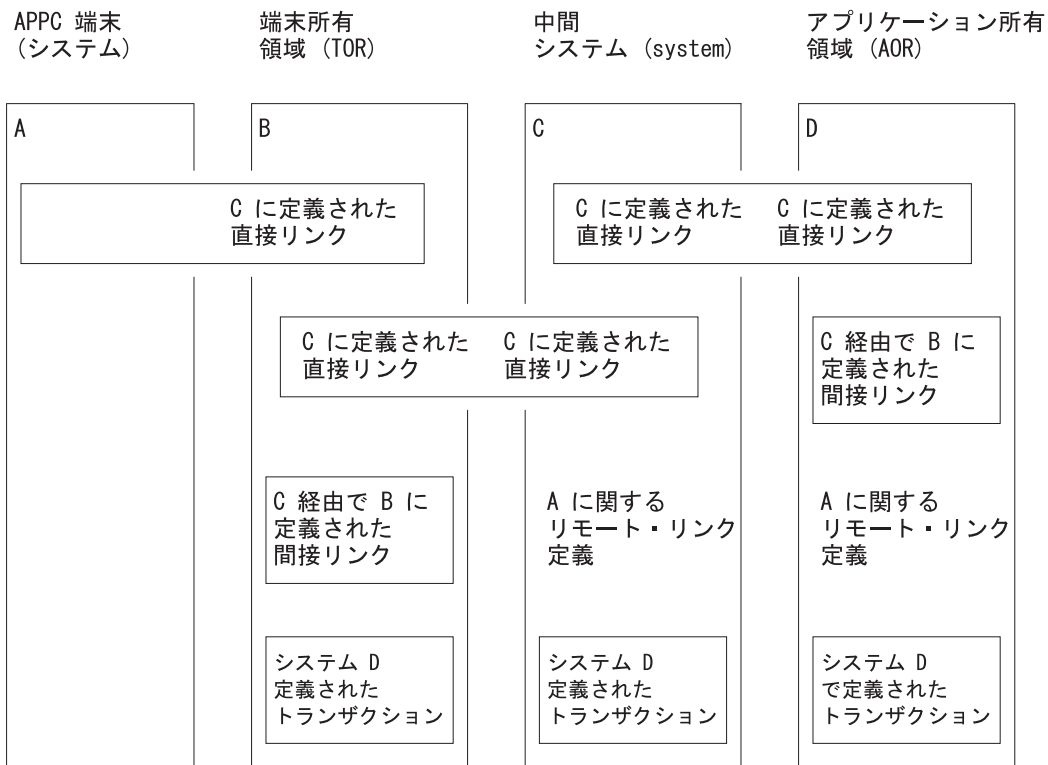
図 29. デイジー・チェーンされたシステムを介した APPC 端末へのトランザクション・ルーティング
