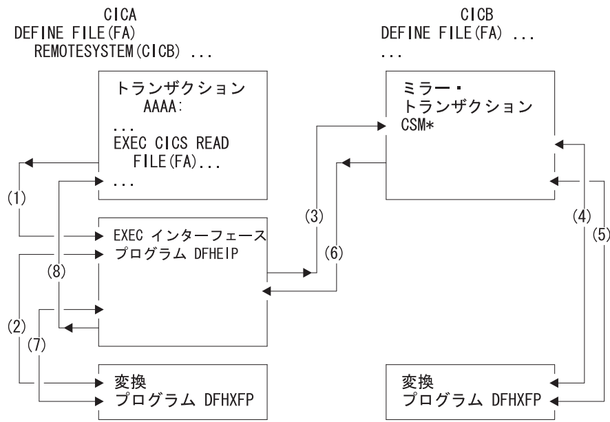
図9. 機能シップにおける変換プログラムとミラー
