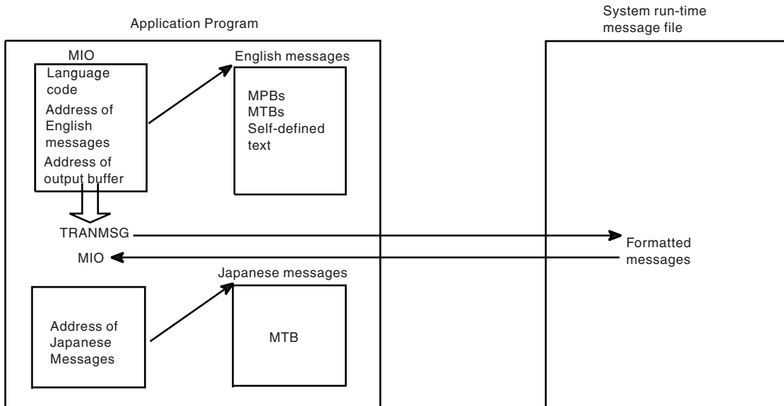
Figure 22-9. Using the TRANMSG Macro
