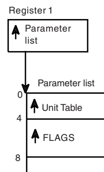
Figure A-1. Input Parameter List
