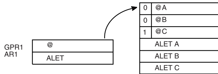
Figure 2-5. AR Mode Parameter List
