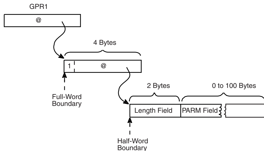
Figure 2-4. Primary Mode Parameter List
